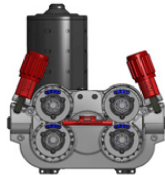
Drahtvorschubgetriebe SF ST4
