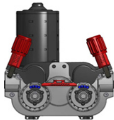
Drahtvorschubgetriebe SF SS4
